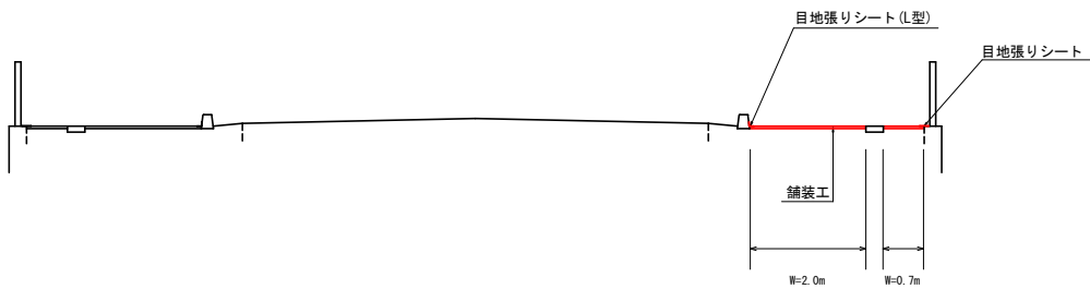
目地張りシート(L型) S=1:5
