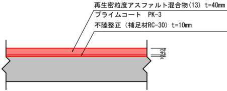
舗装構成 non scale
