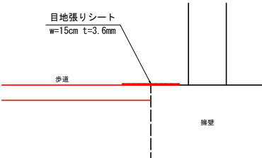
目地張りシート S=1:5
